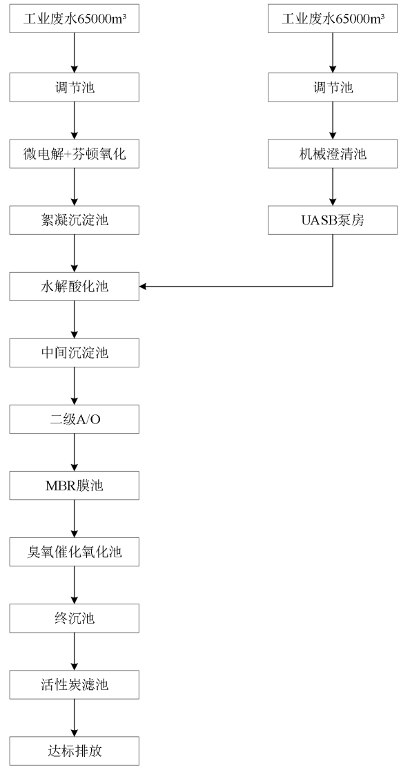
图 5.3-2 提标改造后的污水处理工艺流程图
